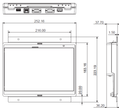
PFXGP4502WADWR(带安装托架)
